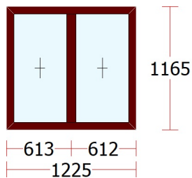
Fereastră19 - 1 buc.
