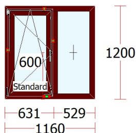
Fereastră06 - 1 buc.
