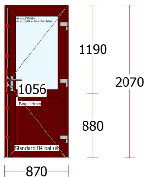
Ușă27 - 1 buc.
