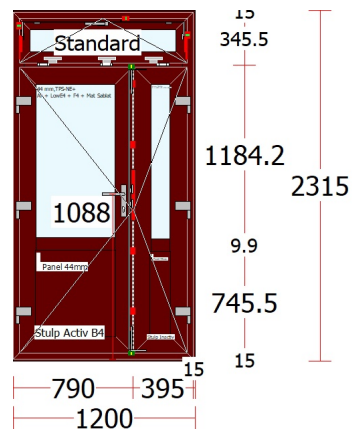
Ușă28 - 1 buc.
