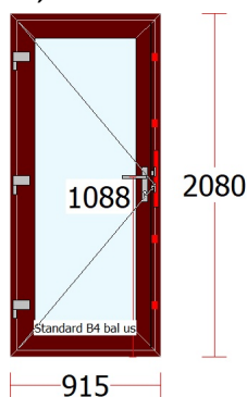
Ușă08 - 1 buc.
