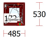
Fereastră14 - 1 buc.
