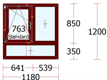
Fereastră04 - 1 buc.
