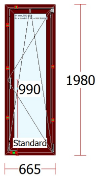
Ușă25 - 1 buc.
