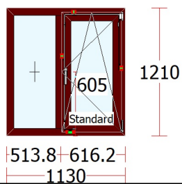
Fereastră19 - 1 buc.
