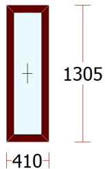
Fereastră15 - 1 buc.
