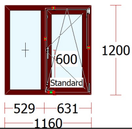
Fereastră13 - 1 buc.
