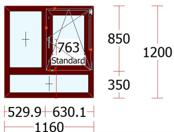
Fereastră03 - 1 buc.
