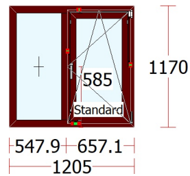
Fereastră22 - 1 buc.
