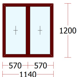
Fereastră09 - 1 buc.
