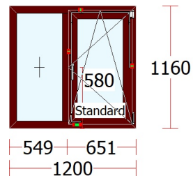
Fereastră24 - 1 buc.
