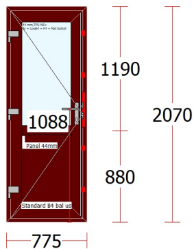
Ușă25 - 1 buc.
