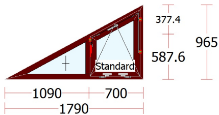
Fereastră15 - 1 buc.
