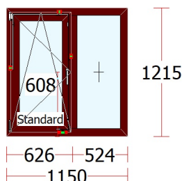
Fereastră10 - 1 buc.
