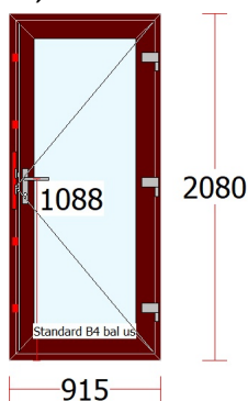
Ușă07 - 1 buc.
