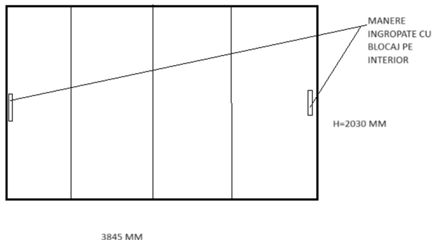
POZITIONARE PANOURI SINA L1
