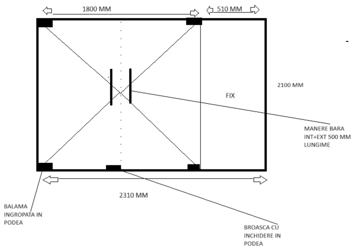
POZITIA NR 2: USA DUBLA, STICLA SECURIZATA CLARA CU BALAMALE INGROPATE CU AMORTIZOR, INCUIETOARE IN PARTEA INFERIOARA+MANERE BARA
