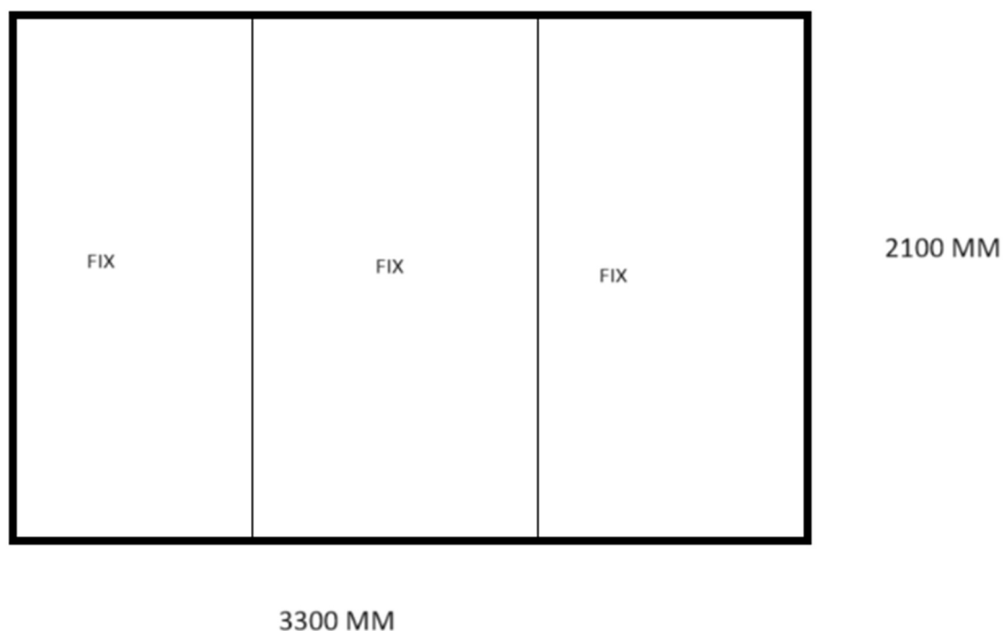
POZITIA NR 1, STICLA SECURIZATA CLARA 10 MM, SINA PERIMETRALA
