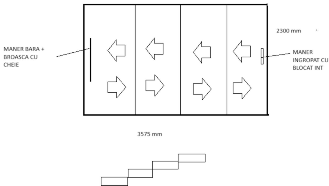
POZITIONARE PANOURI SINA, VEDERE DIN INTERIOR
