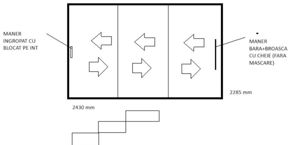
POZITIONARE PANOURI SINA, VEDERE DIN INTERIOR
